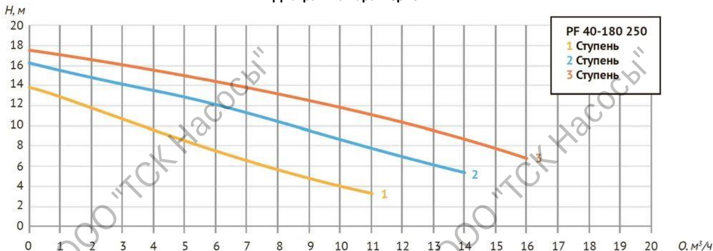
Диаграмма характеристик
