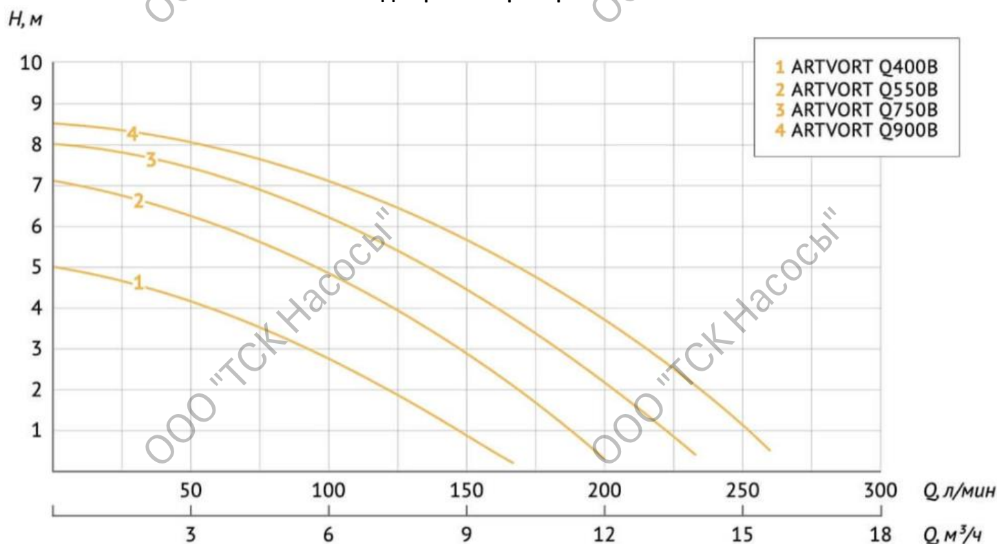
Диаграмма характеристик
