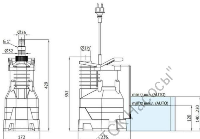
Габаритный чертёж
