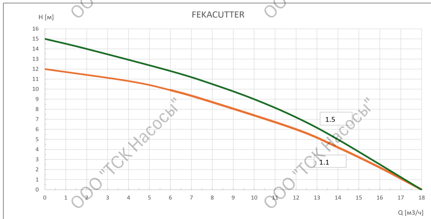
Диаграмма характеристик
