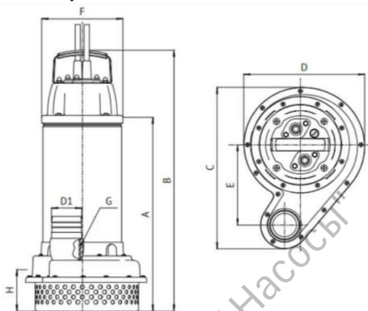
Габаритный чертёж
