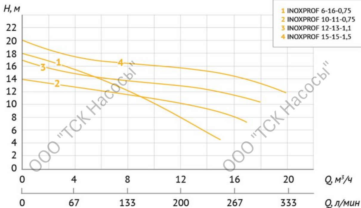
Диаграмма характеристик
