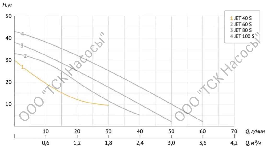
Диаграмма характеристики
