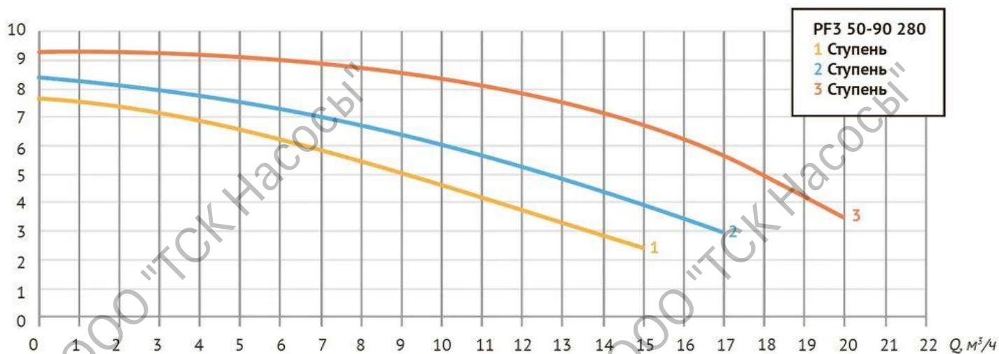
Диаграмма характеристик
