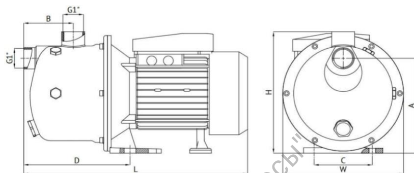
Габаритный чертёж
