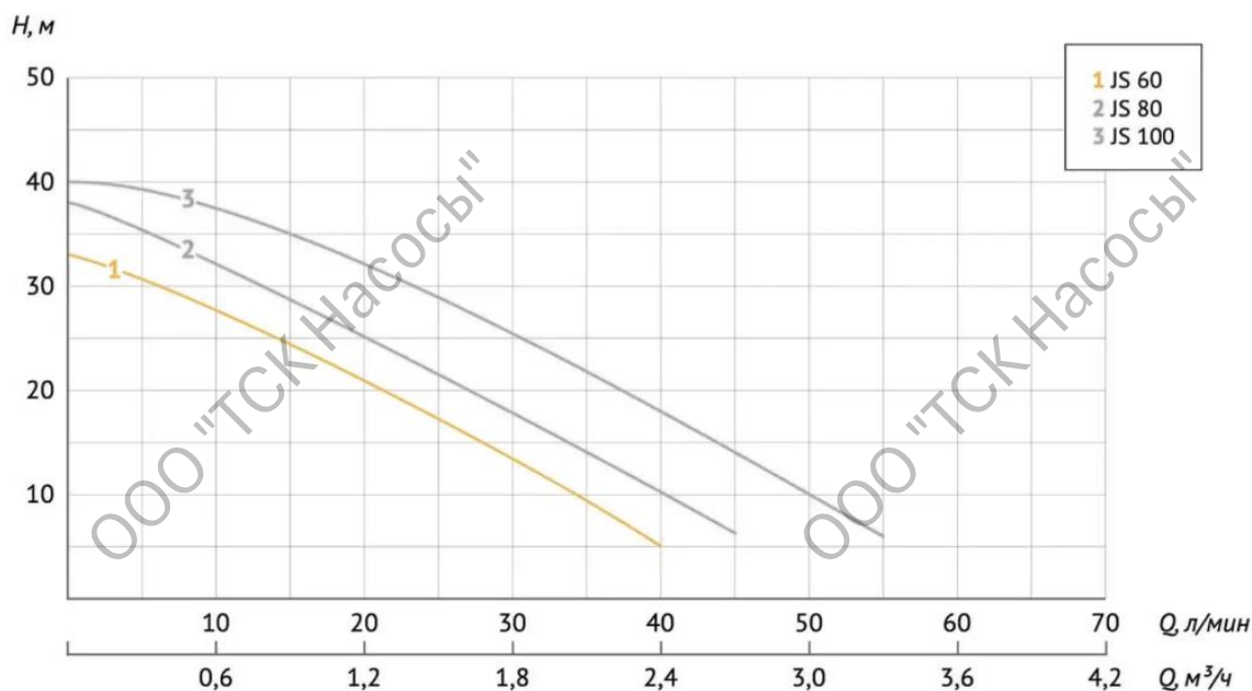
Диаграмма характеристики
