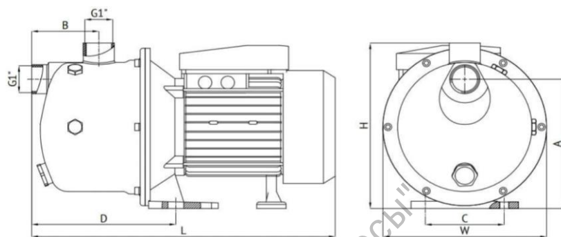
Габаритный чертёж
