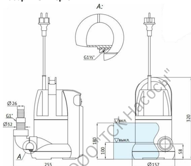
Габаритный чертёж
