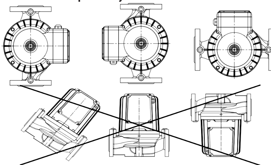
Рисунок 1. Допустимые, и не допустимые положения насоса на трубопроводе
