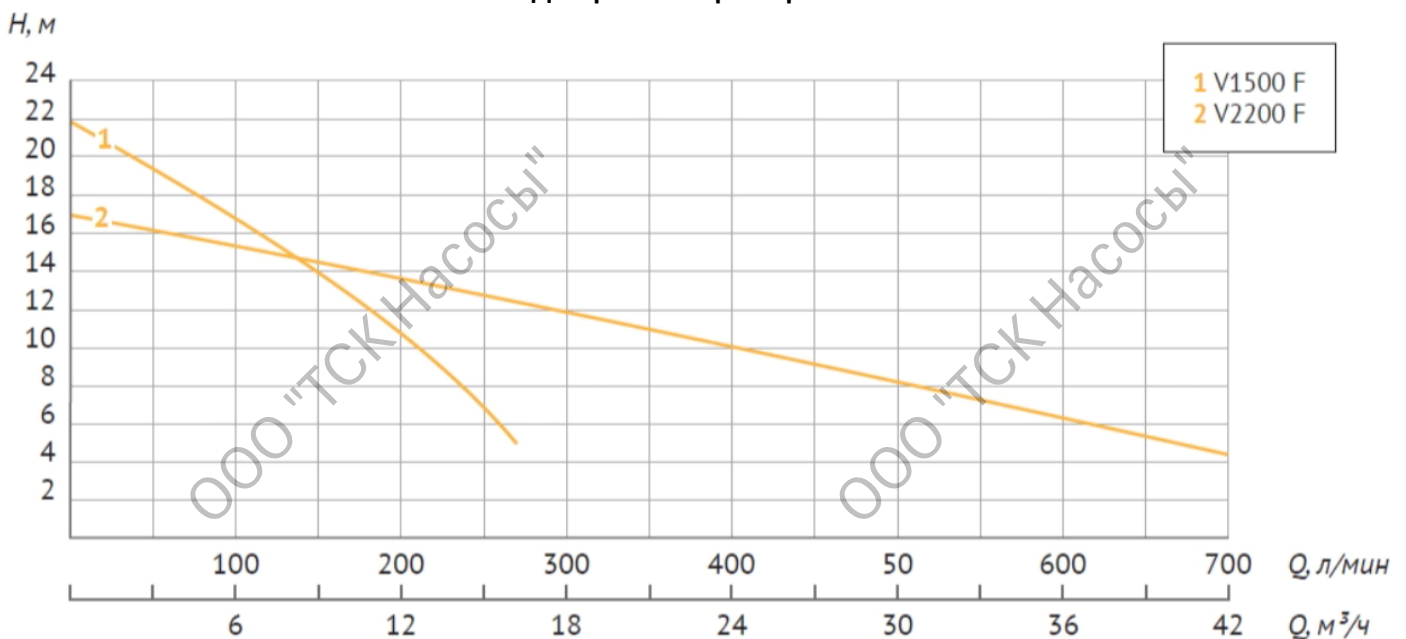
Диаграмма характеристик
