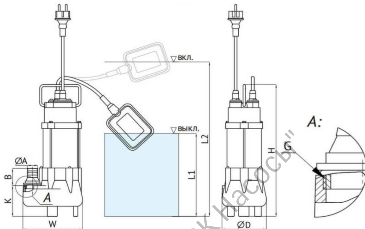
Габаритный чертёж
