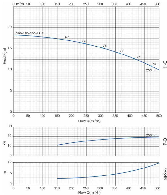
Диаграмма характеристик
