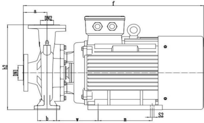
Габаритный чертёж
