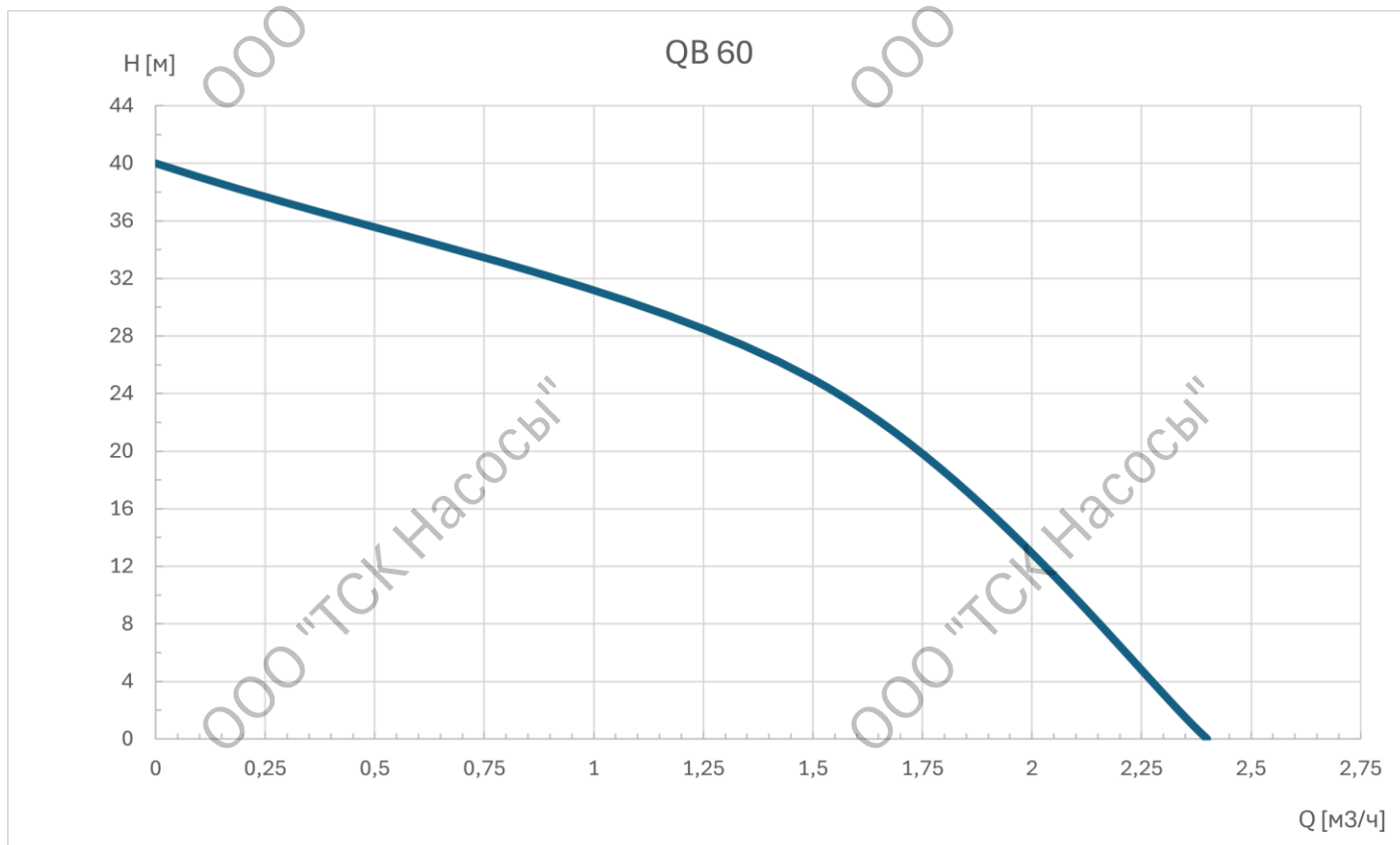
Диаграмма характеристик
