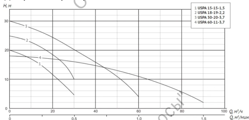
Диаграмма характеристик
