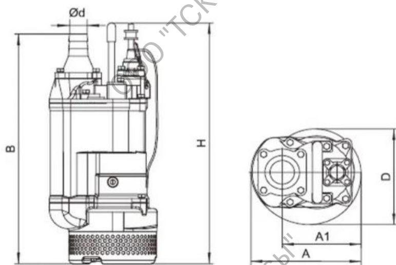
Габаритный чертёж
