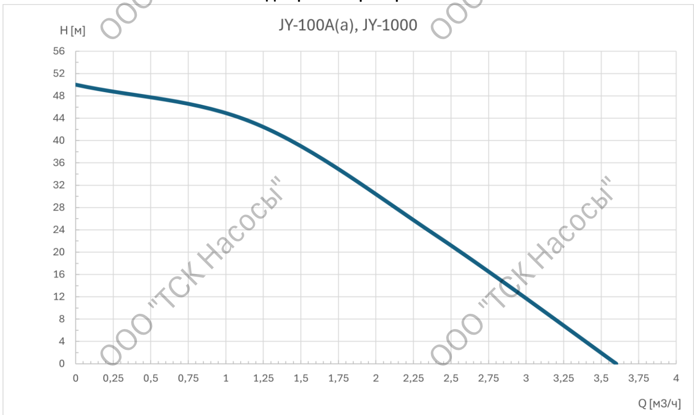
Диаграмма характеристик
