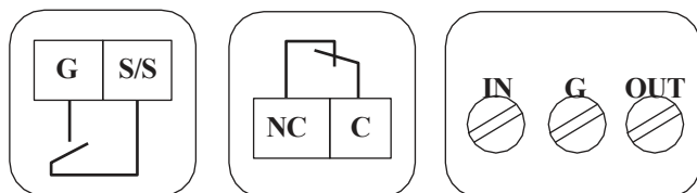
Рисунок 9 – Дополнительные интерфейсы на плате
