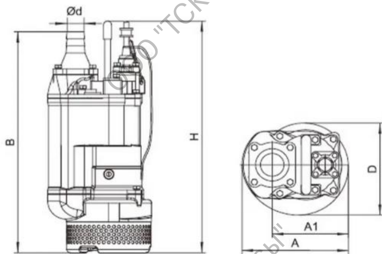
Габаритный чертёж
