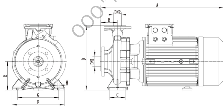
Габаритный чертёж
