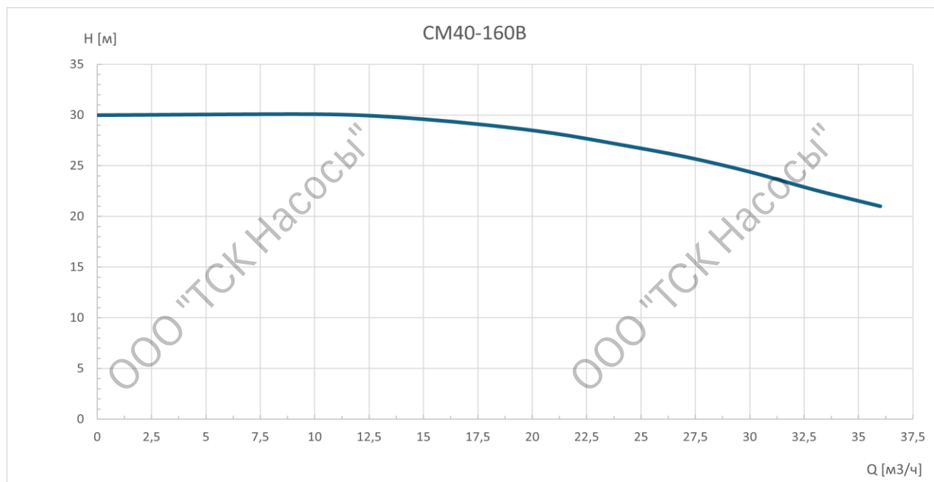
Диаграмма характеристик
