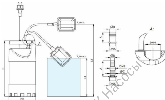
Габаритный чертёж
