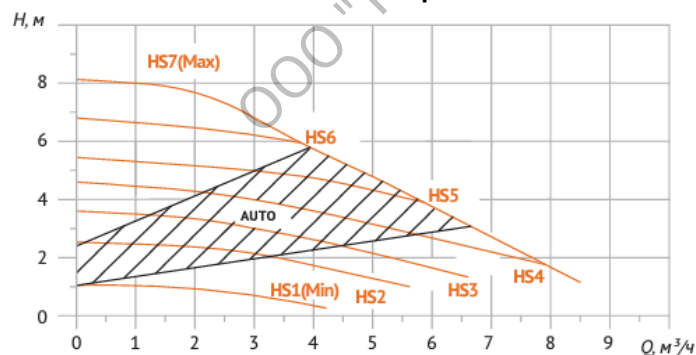
Режим пропорционального давления
