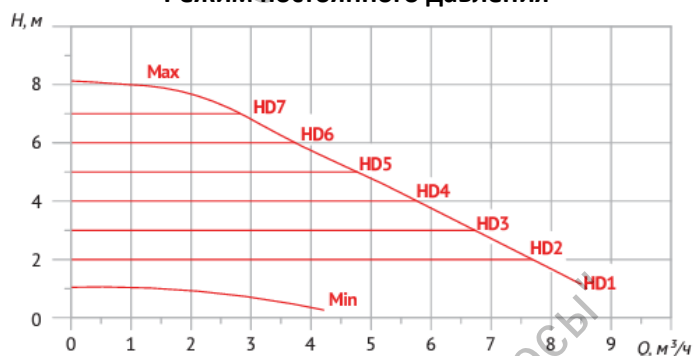
Режим постоянного давления
