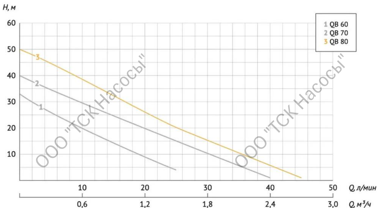
Диаграмма характеристики
