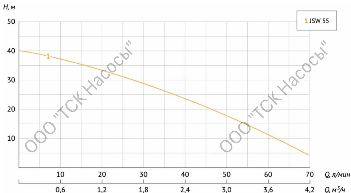
Диаграмма характеристики
