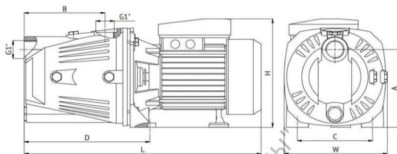
Габаритный чертёж
