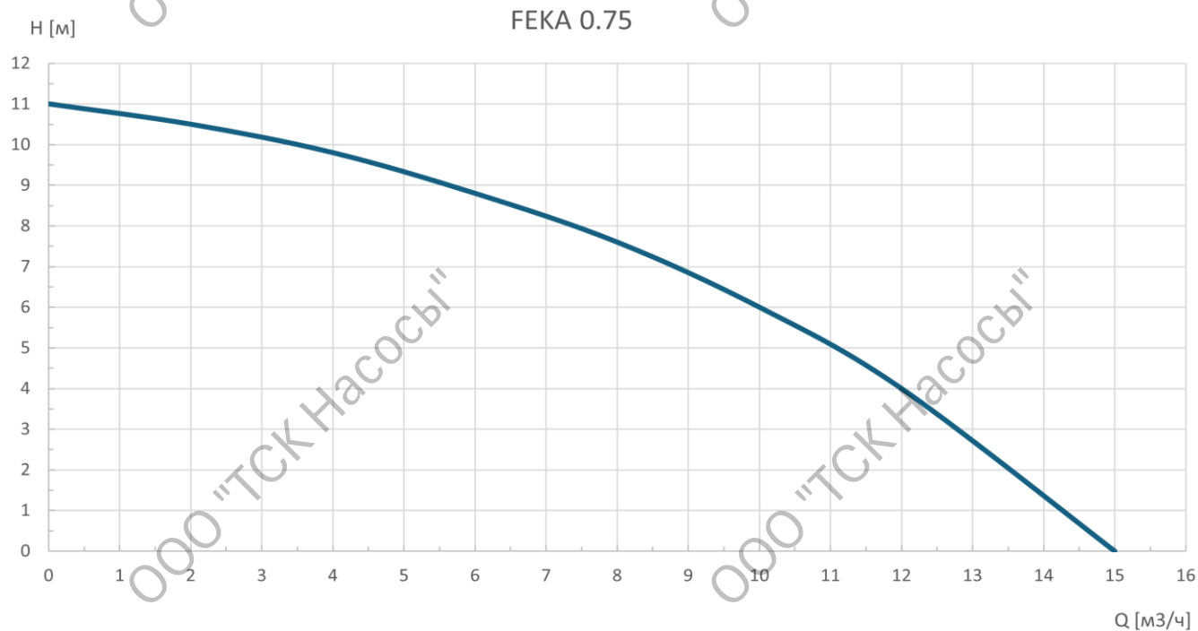
Диаграмма характеристик
