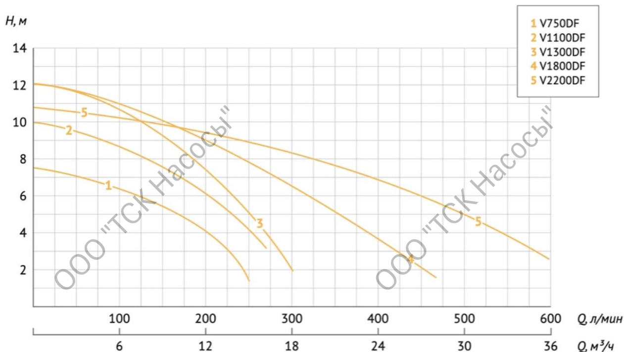
Диаграмма характеристик
