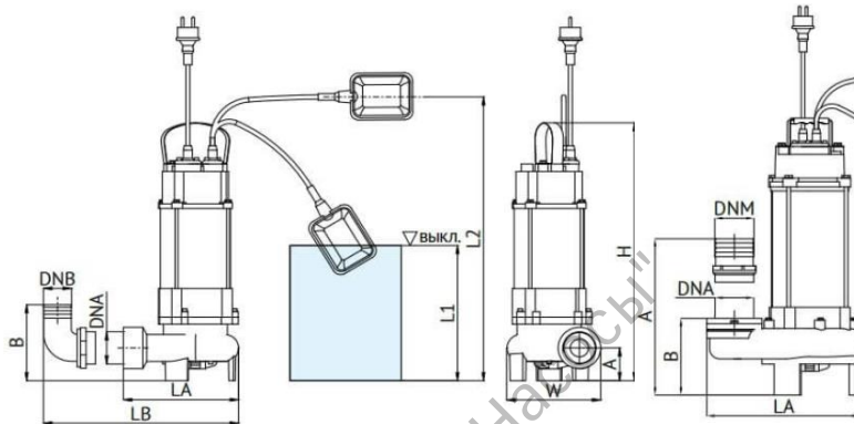
Габаритный чертёж
