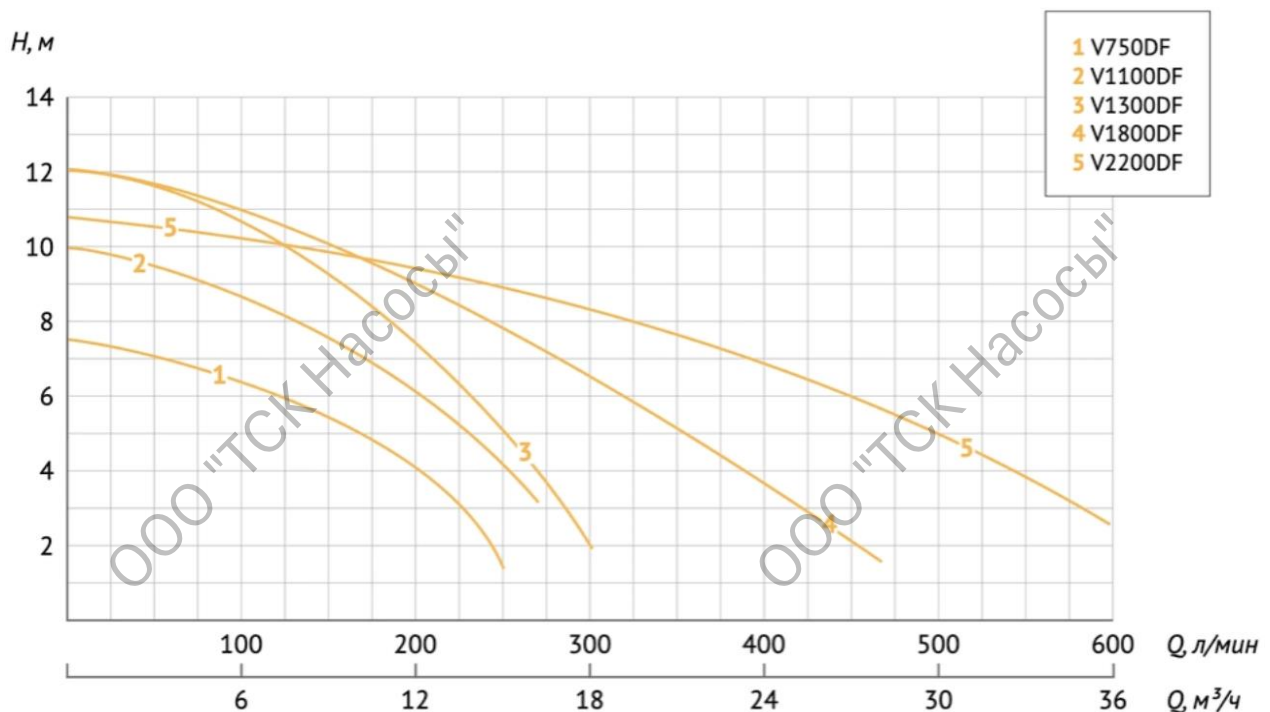
Диаграмма характеристик
