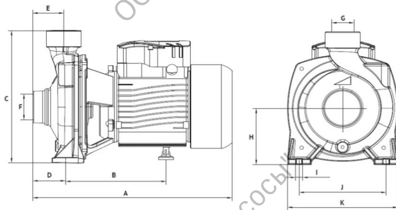
Габаритный чертёж
