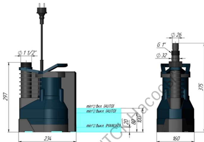
Габаритный чертёж
