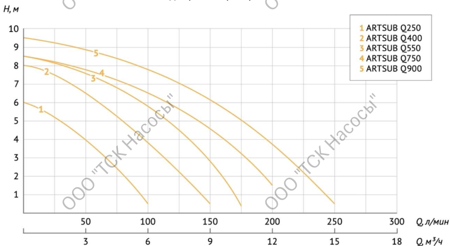
Диаграмма характеристик
