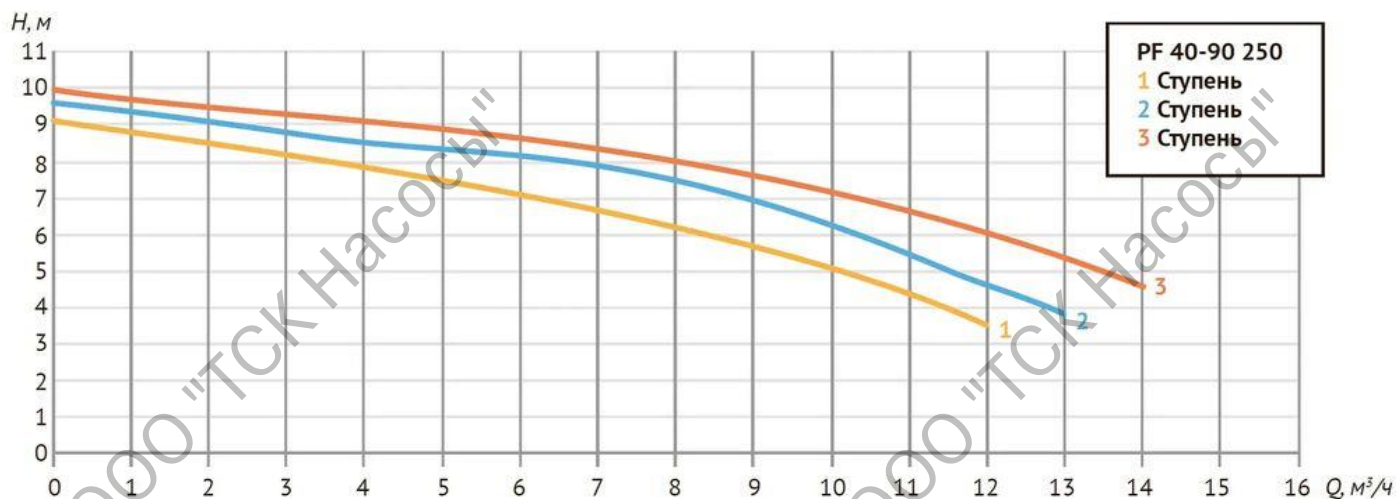
Диаграмма характеристик
