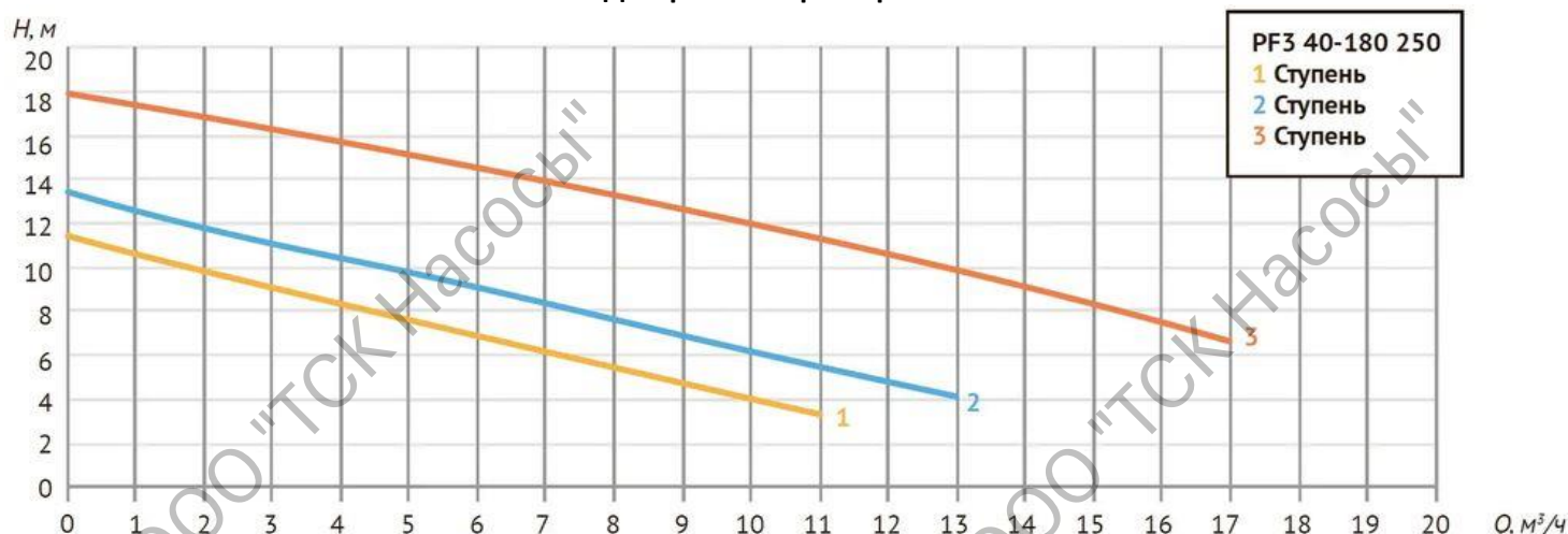
Диаграмма характеристик
