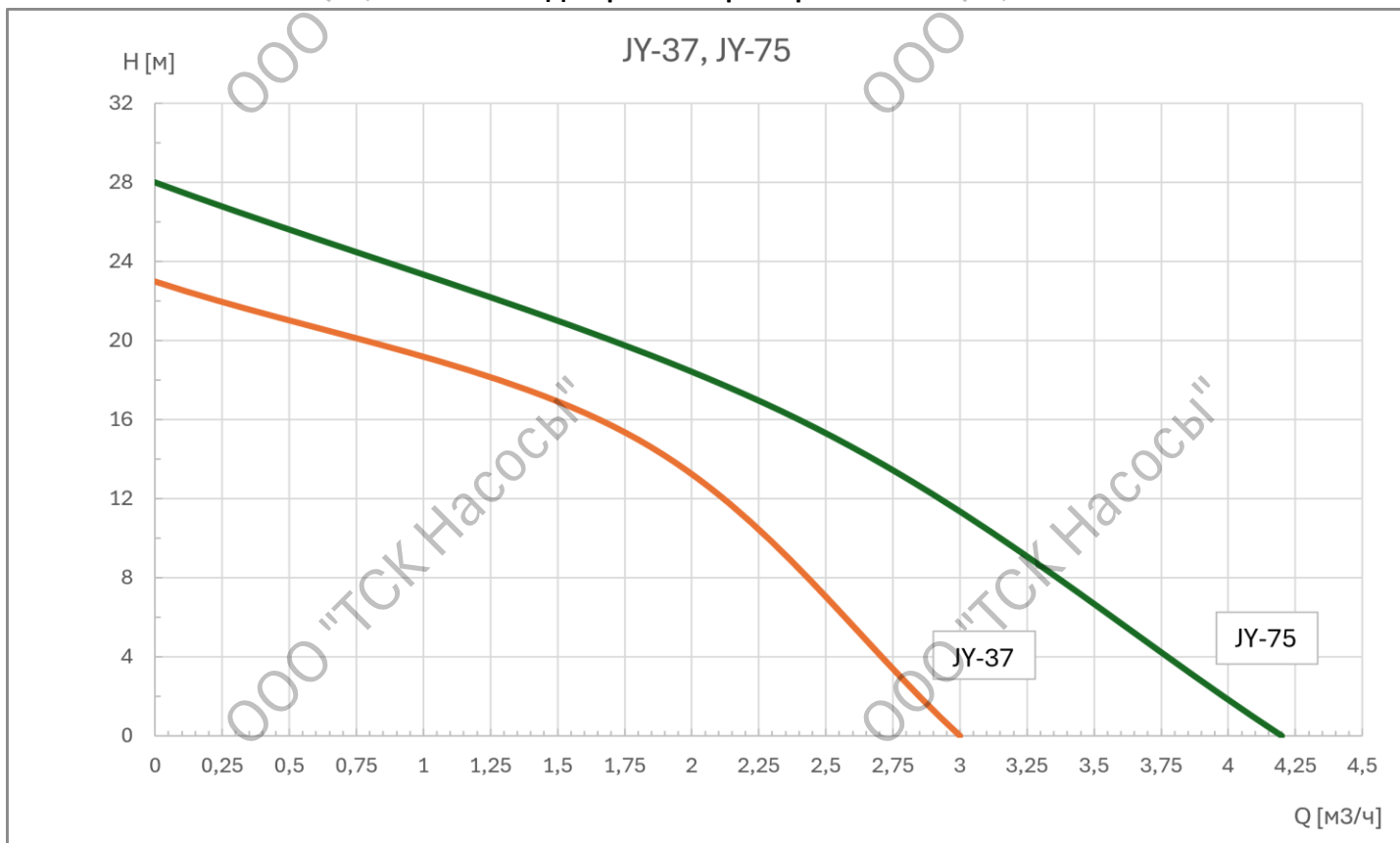
Диаграмма характеристик
