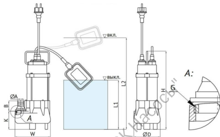
Габаритный чертёж
