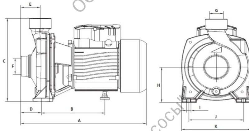
Габаритный чертёж
