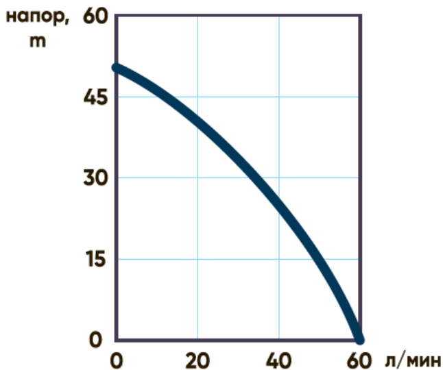
рис 1. Рабочие кривые электронасосов
