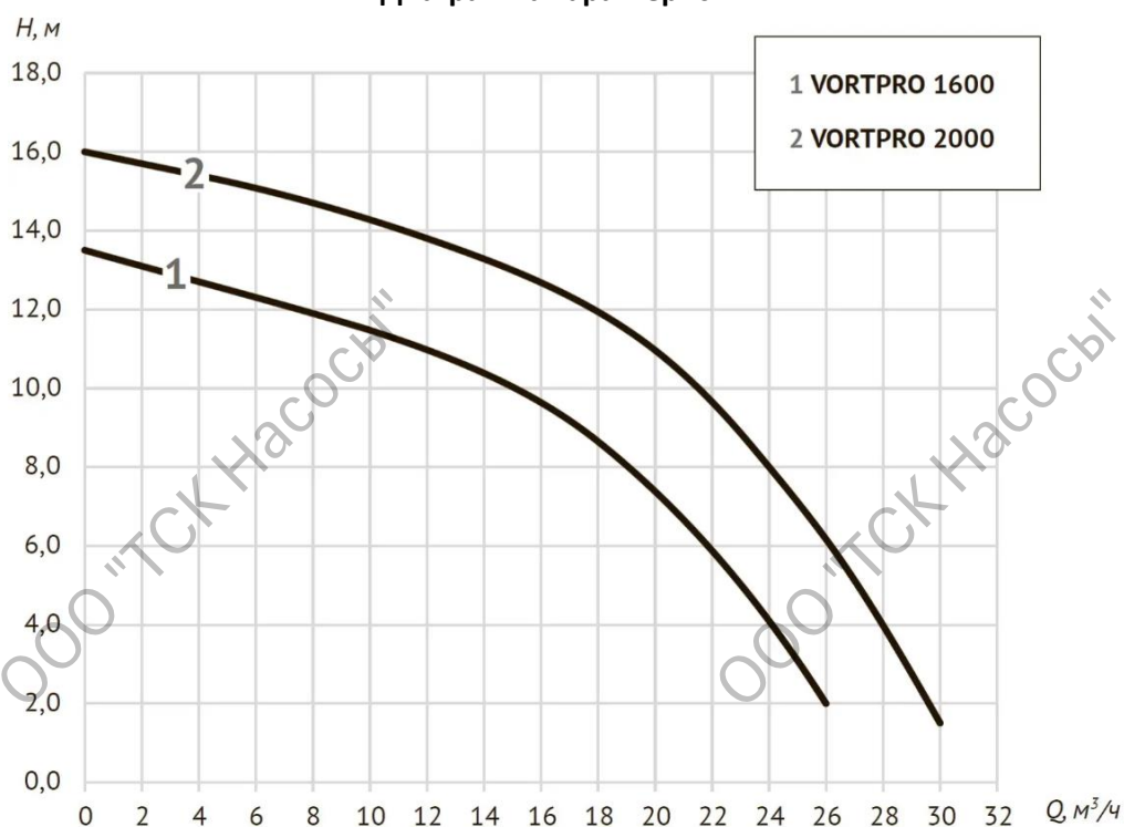
Диаграмма характеристик
