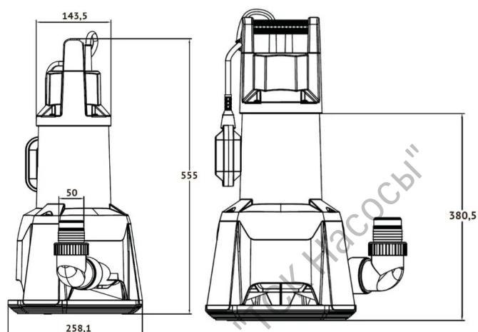
Габаритный чертёж
