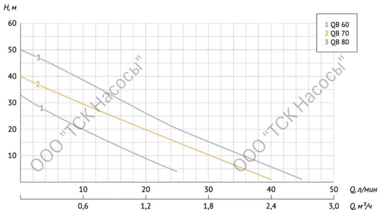
Диаграмма характеристики
