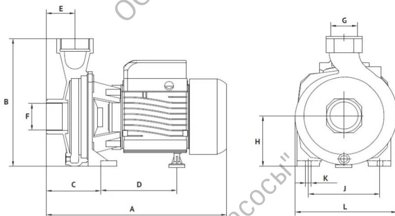
Габаритный чертёж
