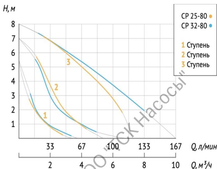
Диаграмма характеристик
