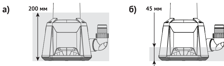
Рисунок 6 – Минимальный уровень воды: а) - для работы насоса, б) - остаточный слой воды
