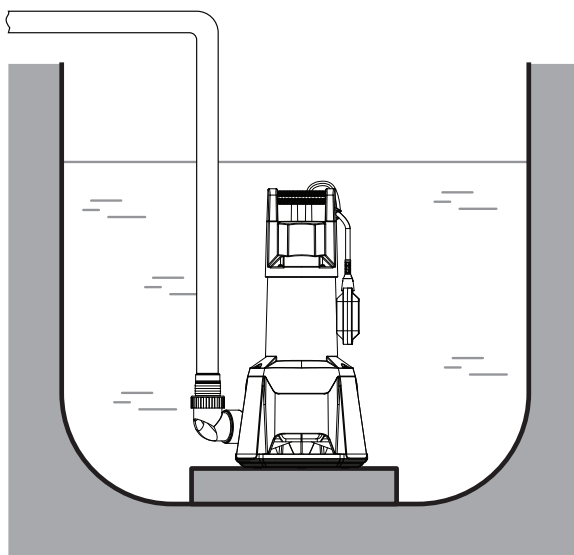
Рисунок 4 – Установка насоса
