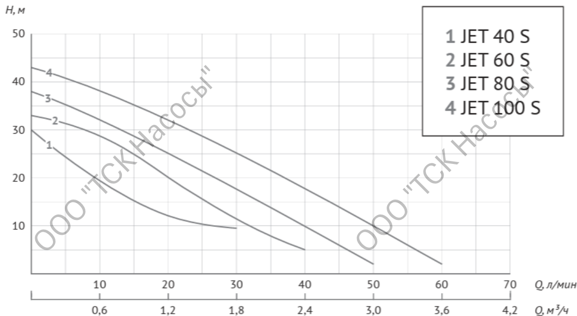
Диаграмма характеристики
