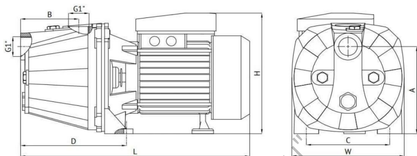
Габаритный чертёж
