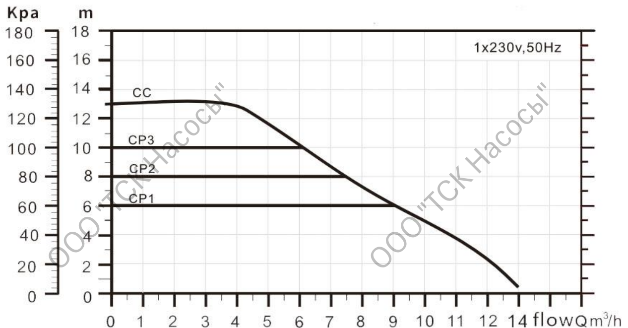
Диаграмма характеристик
