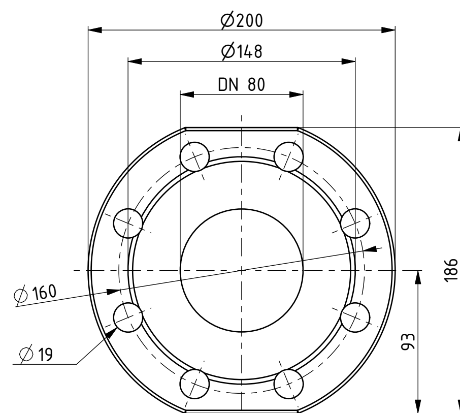
NMTD MAX 80/180-F360 - PN10
