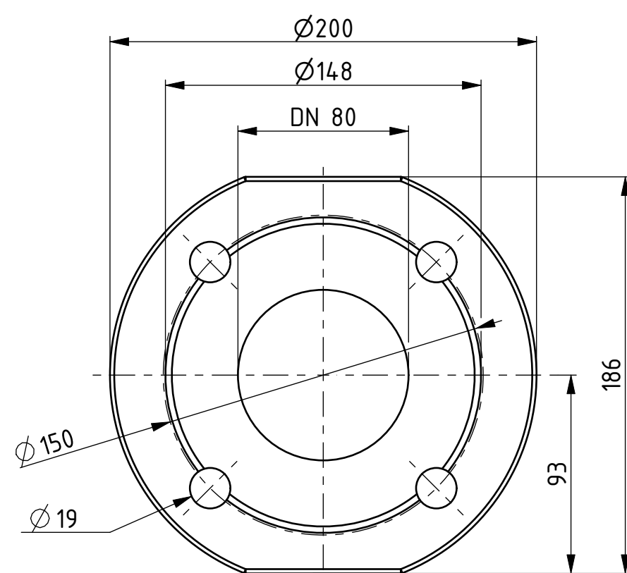
NMTD MAX 80/180-F360 - PN6
