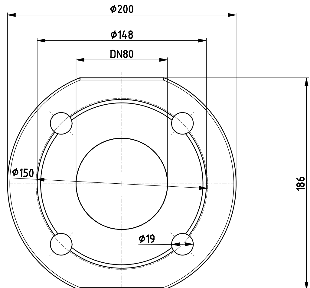
NMTD MAX 80/80-F360 - PN6
