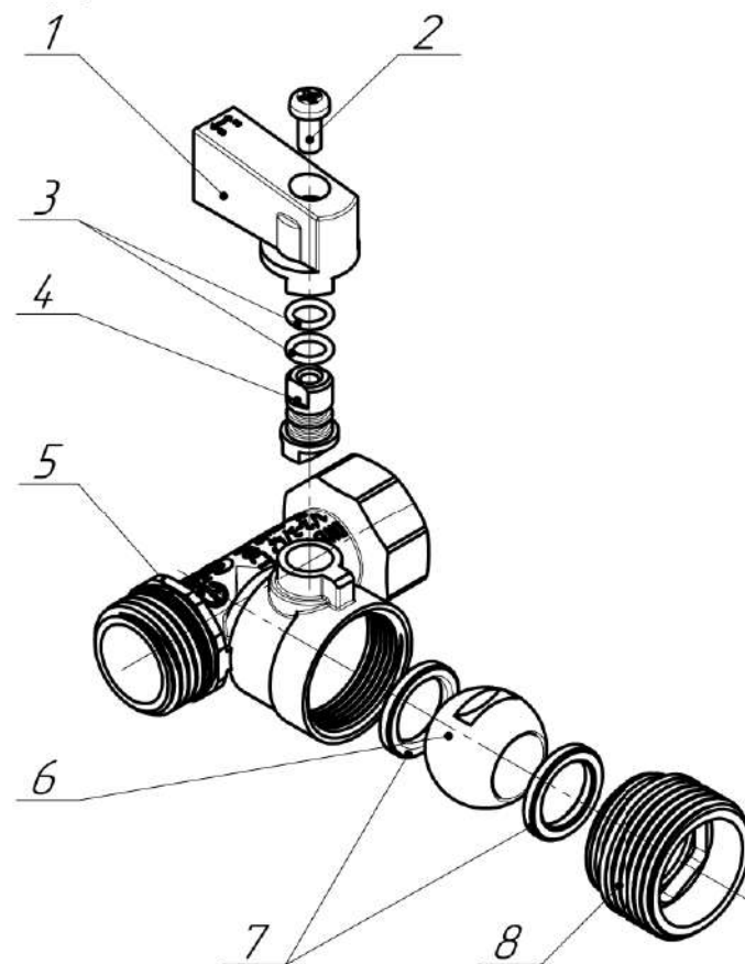
Рисунок 2 – Общий вид и конструкция изделия
