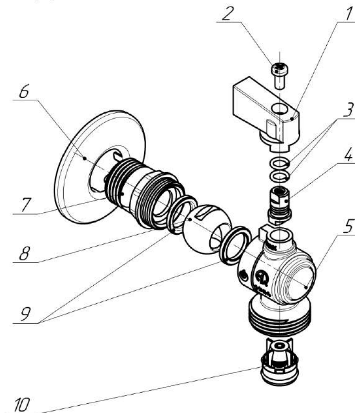
Рисунок 2 – Общий вид и конструкция изделия
