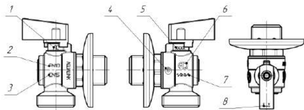
Рисунок 1 – Маркировка на изделии
