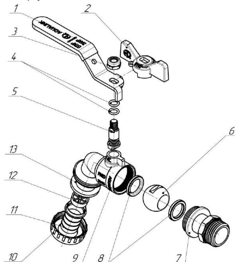
Рисунок 2 – Общий вид и конструкция изделия
