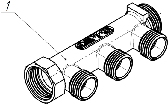
Рисунок 2 – Общий вид и конструкция изделия
