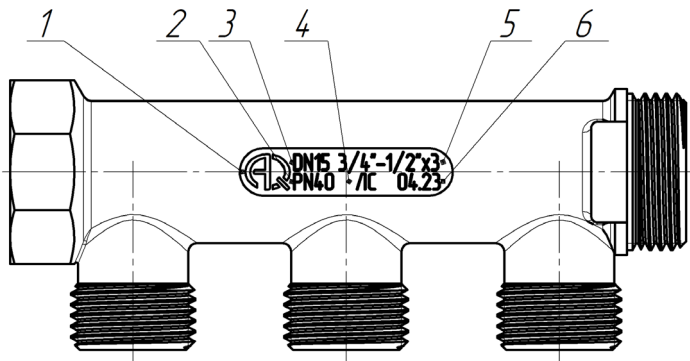
Рисунок 1 – Маркировка на изделии
