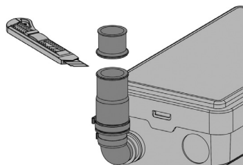
Рисунок 8 – Угловой ступенчатый патрубок КНС
