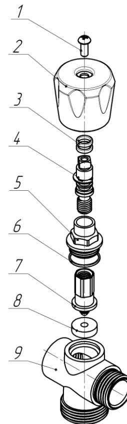
Рисунок 2 – Общий вид и конструкция изделия
