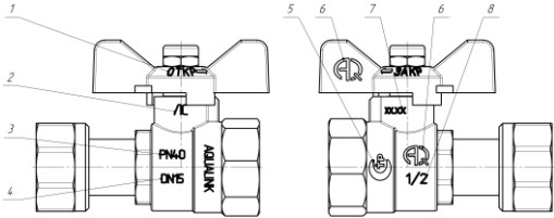
Рисунок 1 – Маркировка на изделии
