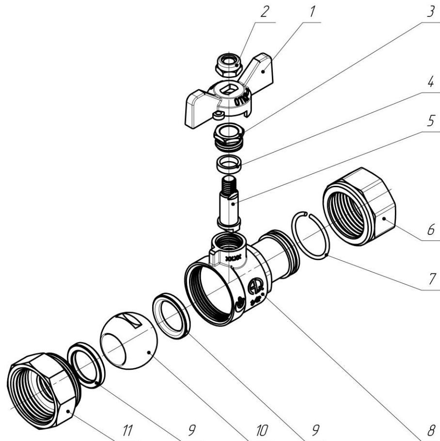
Рисунок 2 – Общий вид и конструкция изделия
